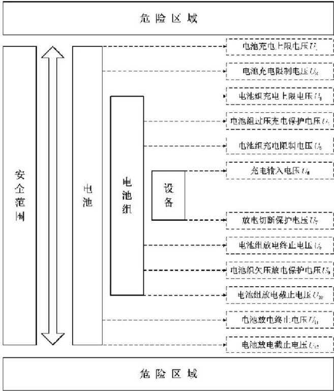
图1 电压管理示意图
