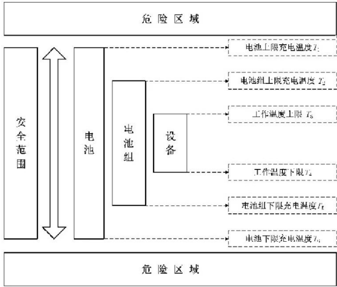
图 3 充电温度管理示意图
