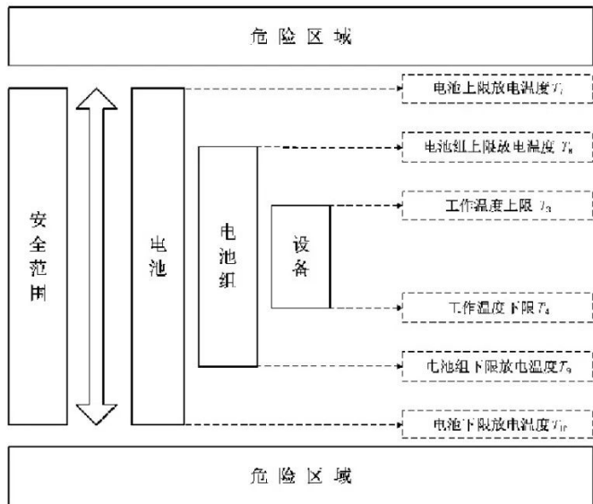
图 4 放电温度管理示意图
